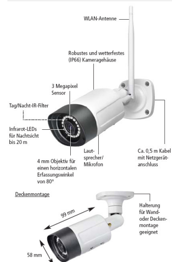
Kamera WR120B4
